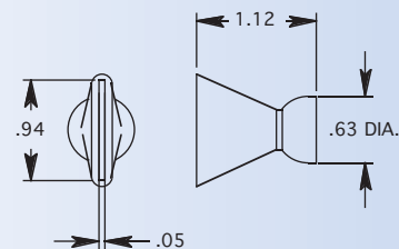
1" FLARE NOZZLE
