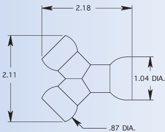
1/2" Y MOLDED
