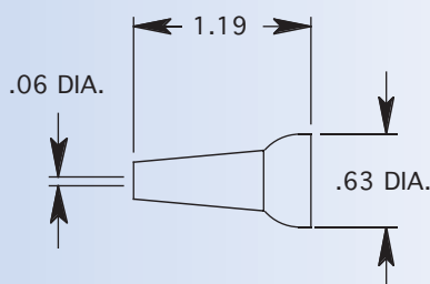
1/16" NOZZLE
