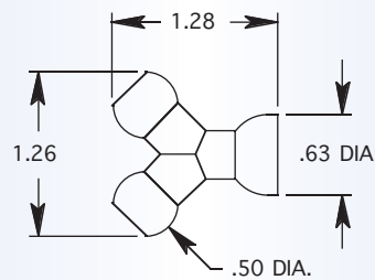
1/4" Y
