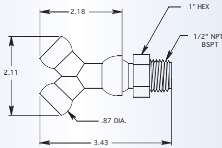
1/2" Y X 1/2" CONNECTOR
